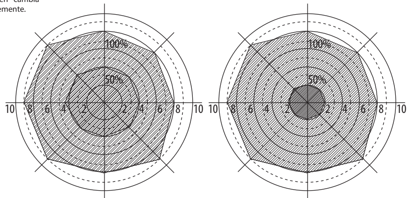
Altura de instalación en el techo: 2,5 m Ajuste del rango de detección: 100%/50%
